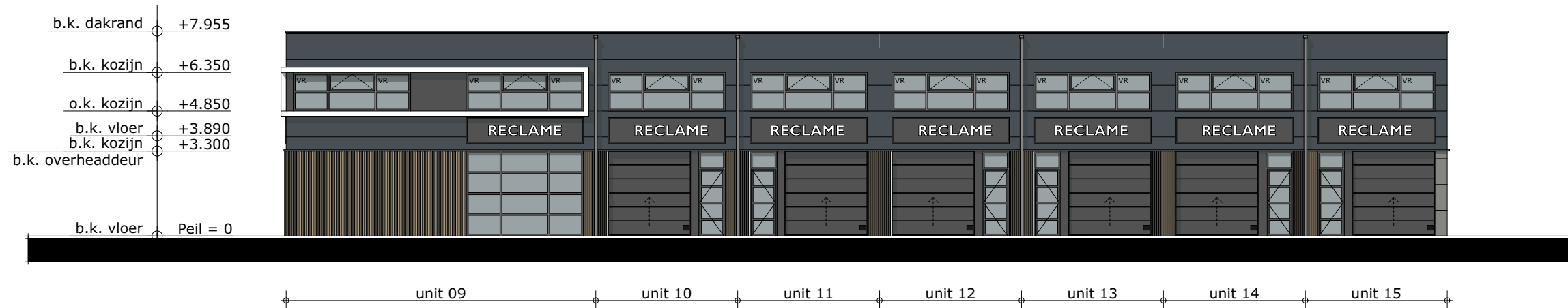
ZUID-OOST GEVEL
