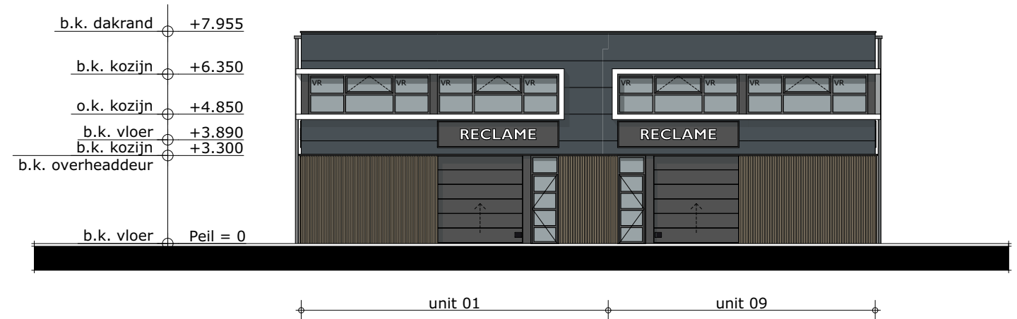
ZUID-WEST GEVEL
