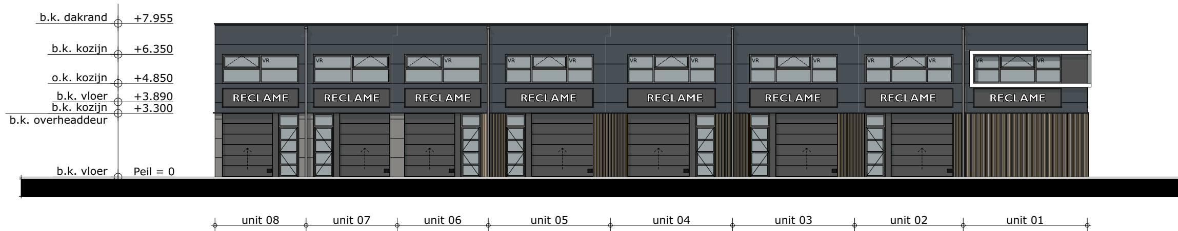
NOORD-WEST GEVEL
