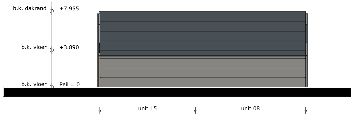
NOORD-OOST GEVEL
