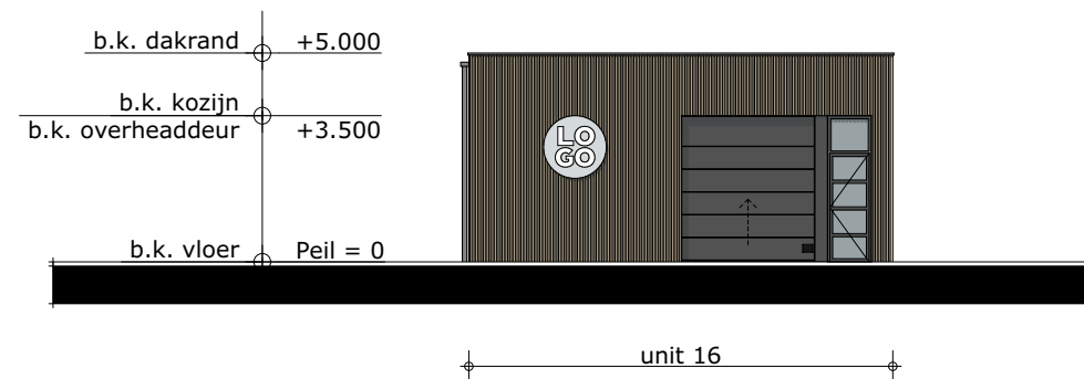
ZUID-WEST GEVEL
